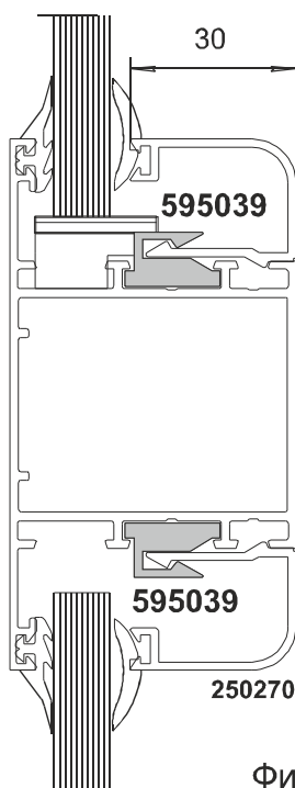
Схема установки 595039
