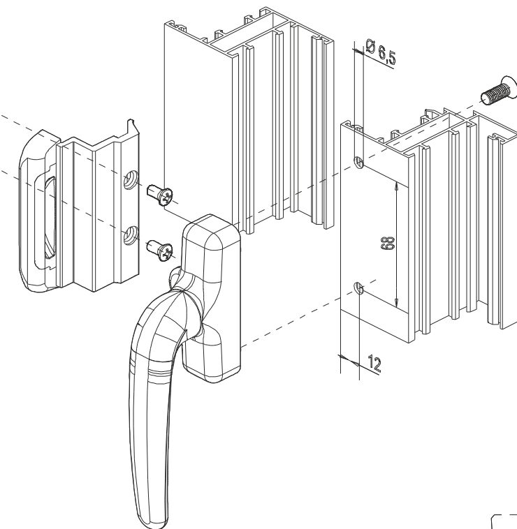
Схема установки ручки 401067
